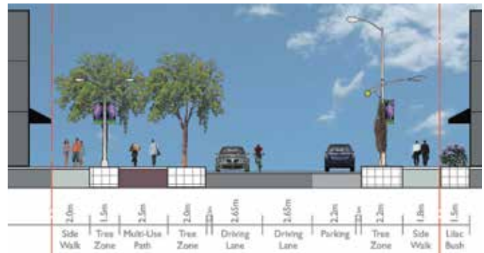
CS-1b: Complete cross-section
